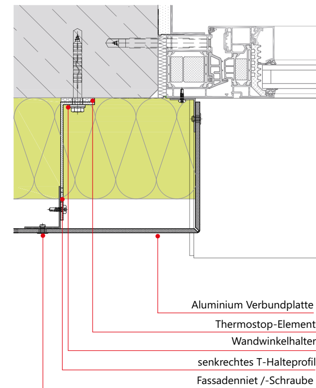
DETAIL FENSTERLEIBUNG VAR. 2
